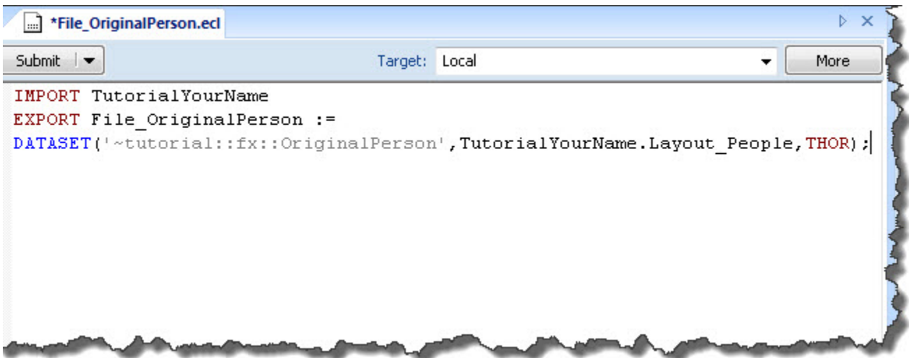
Figure 15. File_OriginalPerson.ecl
