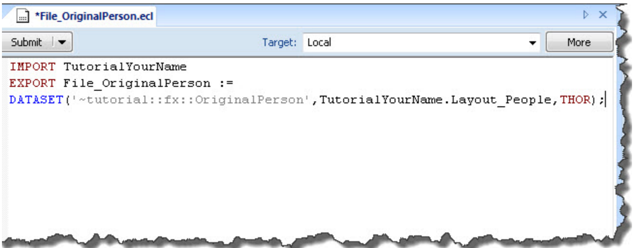
Figure 15. File_OriginalPerson.ecl
